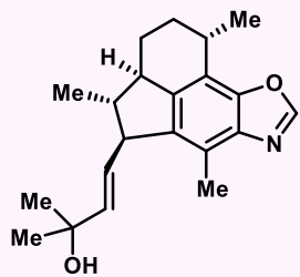
(+)-ileabethoxazole
