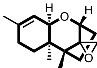
trichothecenes
