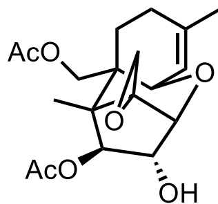
anguidine
