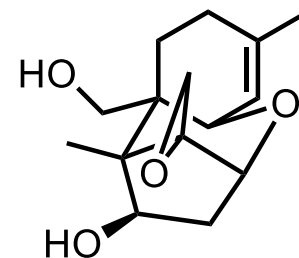
verrucarol
