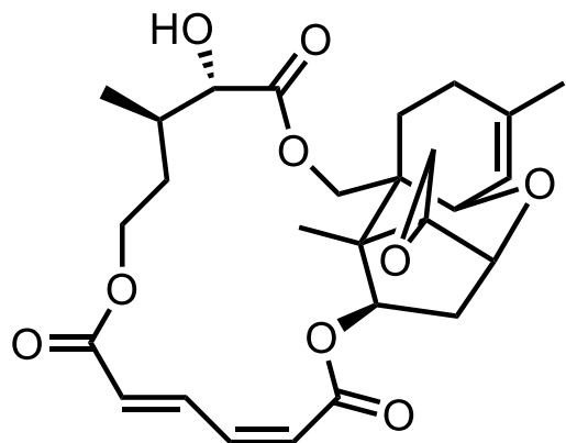
verrucarin A
